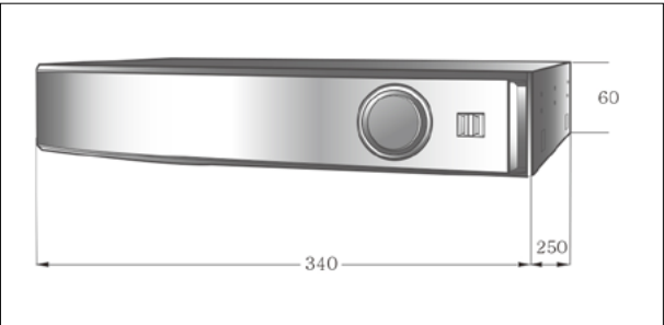
외관도 단위:mm
