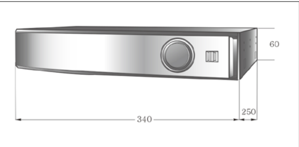
외관도 단위:mm
