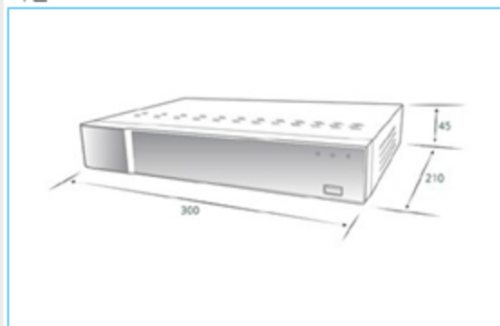
외관도
